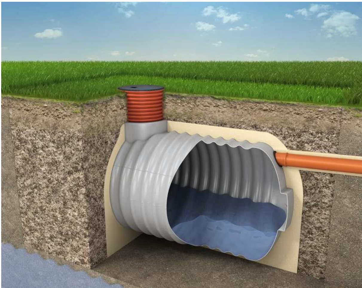
Obr. 1: Montáž nádrže v suchej zemine
