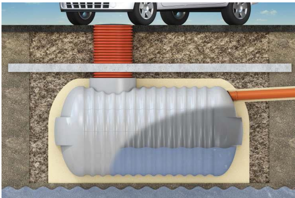
Obr. 4: Správne prevedenie betónovej platne 2
