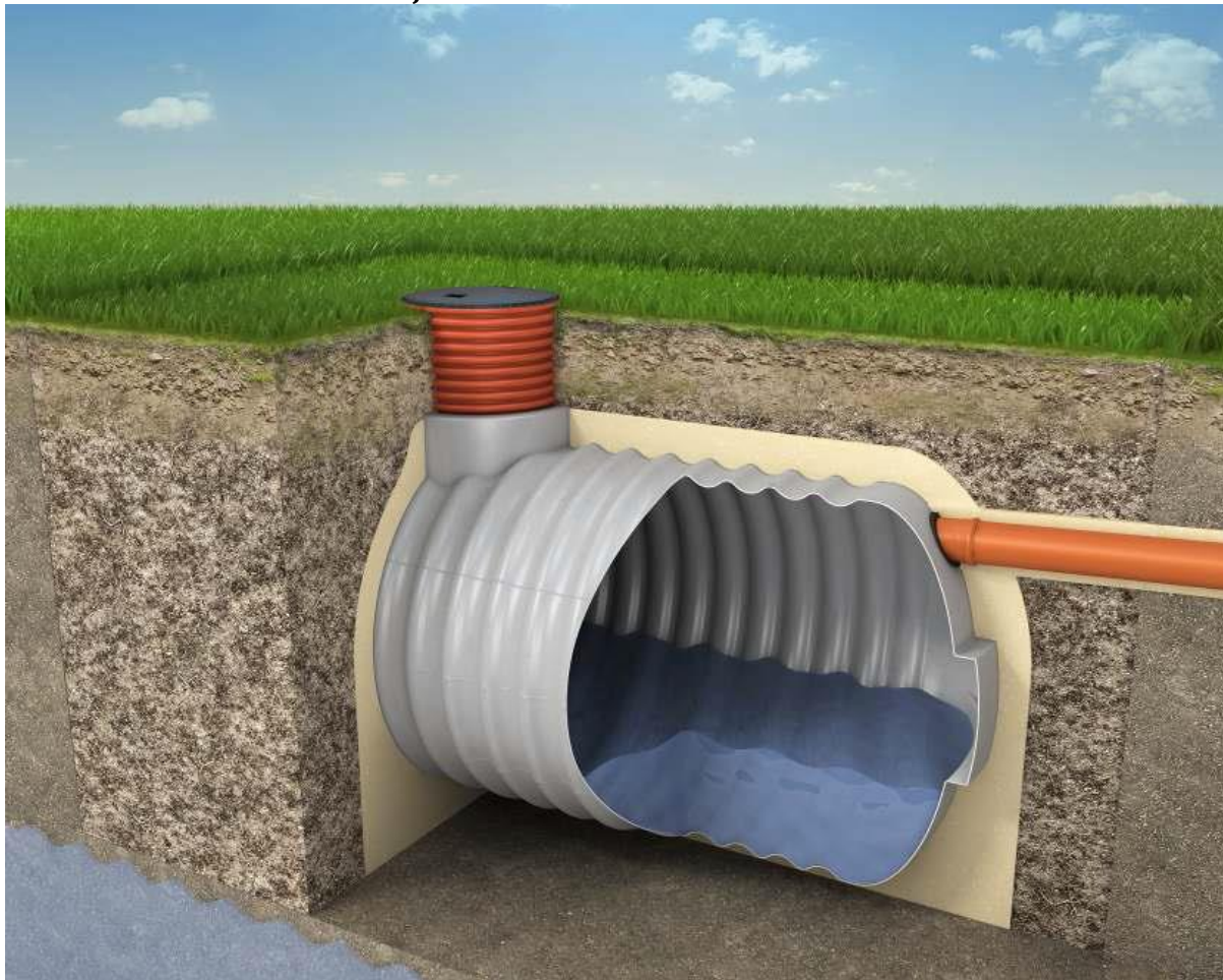
Obr. 1: Montáž nádrže v suchej zemi
